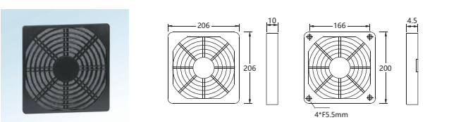
GP-166H(B) for 200mm fan
