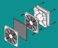
GP-40H(B) for 50mm fan
